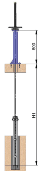
Стандартная колонна
