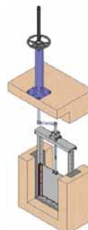
Карданное сочленение
